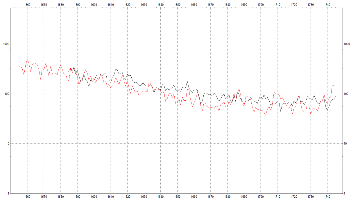
Joonis 2. Eliisabeti kiriku tornivöö männitalade keskmine 2epelt02 (proovid 1+2+3) sünkroonses positsioonis sama kiriku vanema osa pikihoone katusetalastiku keskmisega eli2avg . Kattuvus 161 aastat, TV = 20,3.
