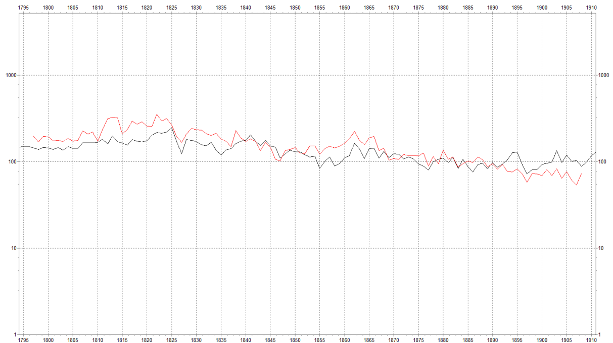
Joonis 4. Eliisabeti kiriku torni kuusepuidust postide keskmine aastarõngalaiuste rida 2eselt04 (proovid 5+6+7+8+9) sünkroonses positsioonis Eesti kuusekronoloogiaga 3esest01 . Kattuvus 112 aastat, TV = 16,4.
