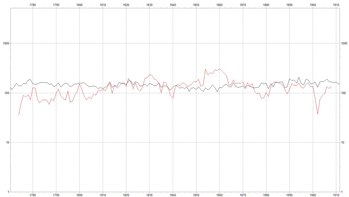
Joonis 3. Eliisabeti kiriku torni männipuidust postide keskmine aastarõngalaiuste rida 2epelt01 (proovid 10+11+12) sünkroonses positsioonis Eesti männikronoloogiaga 3epestcr . Kattuvus 135 aastat, TVH = 6,0.
