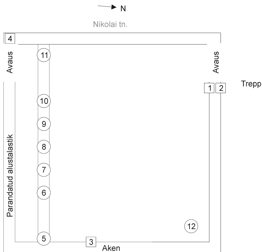
Joonis 1. Puuritud talade (ruudud) ja postide (ringid) asukohad Eliisabeti kiriku tornis.
